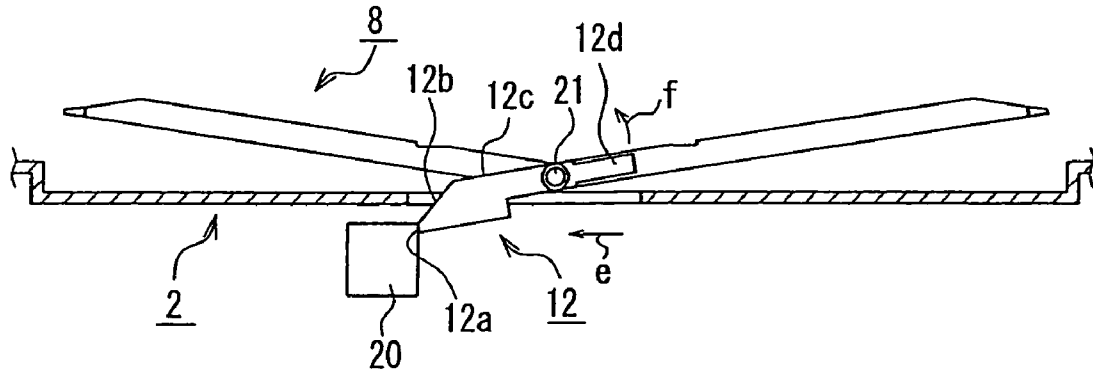
FIG. 10A
