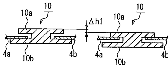
FIG. 16B
