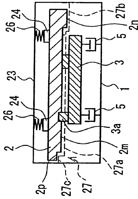
FIG. 31B
