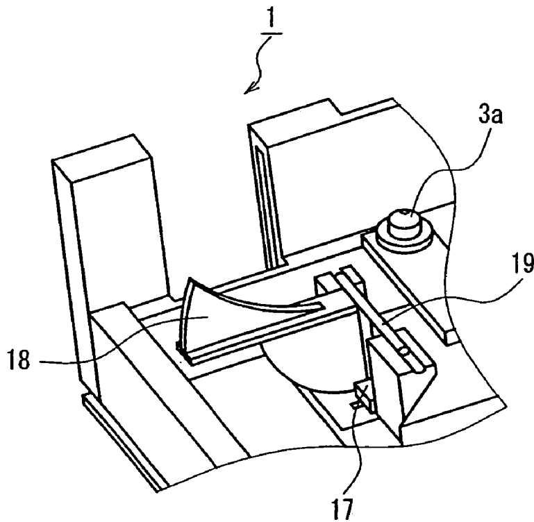
FIG. 23B
