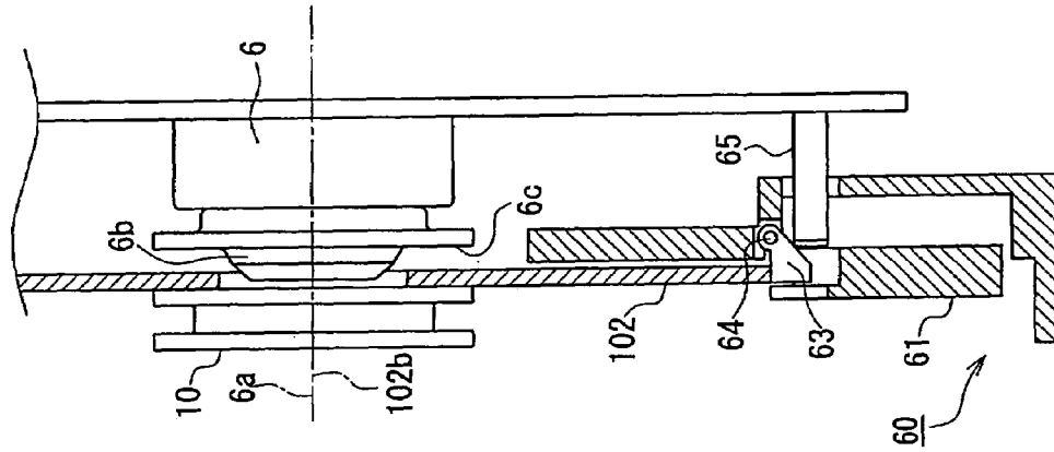
FIG. 26B
