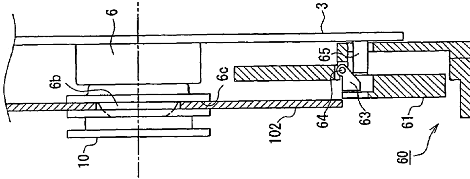
FIG. 26C
