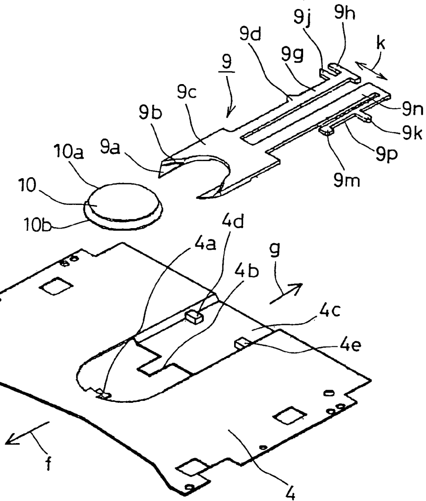
FIG. 16A
