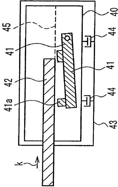
FIG. 31C
